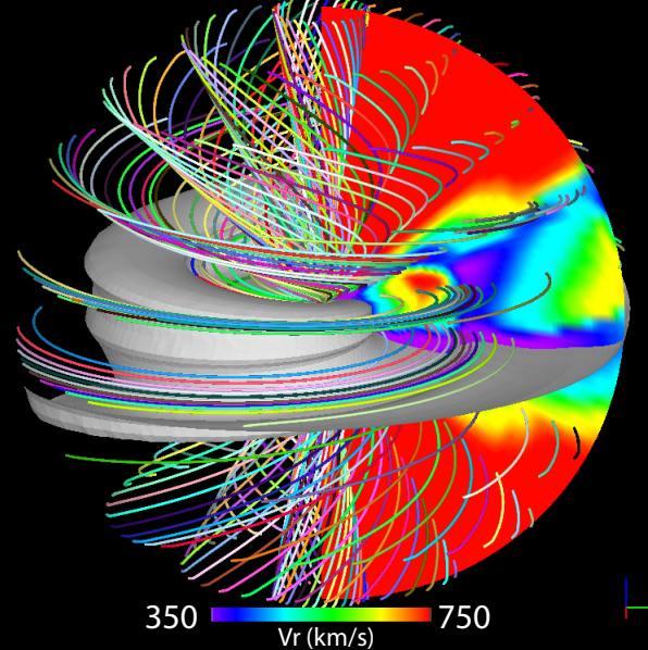
(d) Whole Heliosphere Interval: Heliosphere
